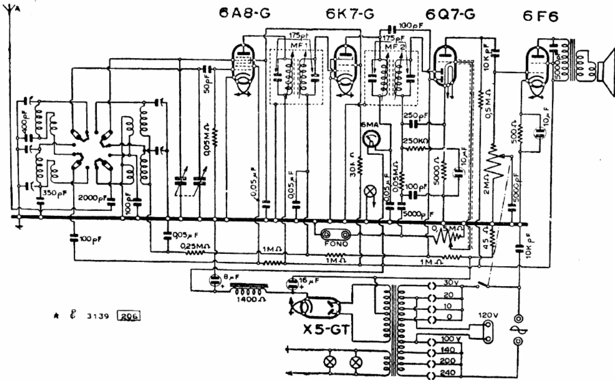
Lo schema elettrico del mod. "501", Sire (telato 2521).
